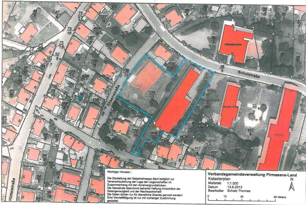
Lageplan
